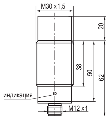
Габаритный чертеж
