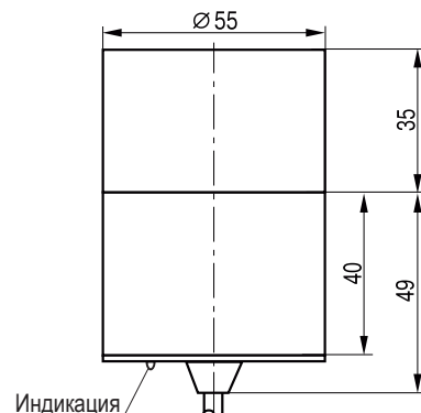
Габаритный чертеж
