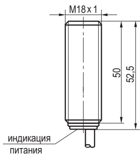
Габаритный чертеж
