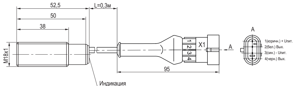
Габаритный чертеж
