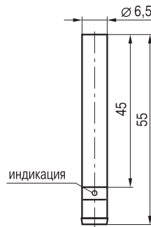
Габаритный чертеж
