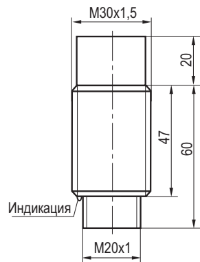
Габаритный чертеж
