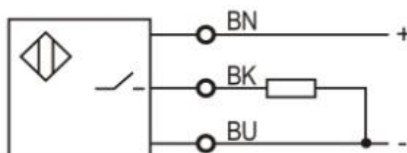
PNP NO
