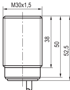
Габаритный чертеж
