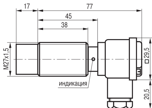
Габаритный чертеж
