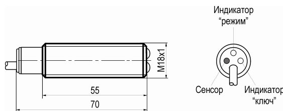
Рисунок 1 - Габаритный чертёж
