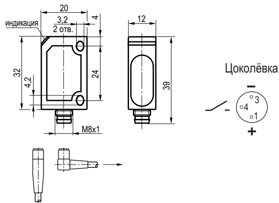
Габаритный чертеж.
