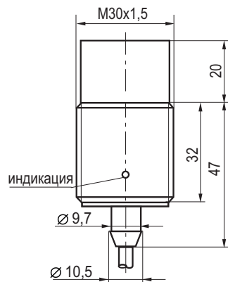
Габаритный чертеж
