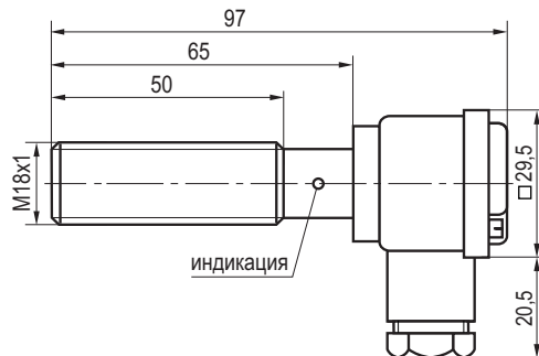
Габаритный чертеж
