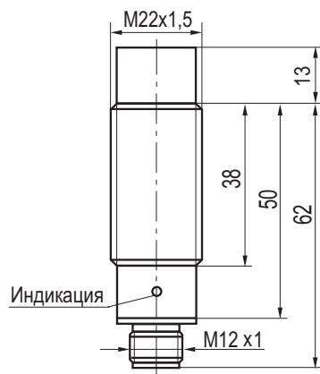
Габаритный чертеж
