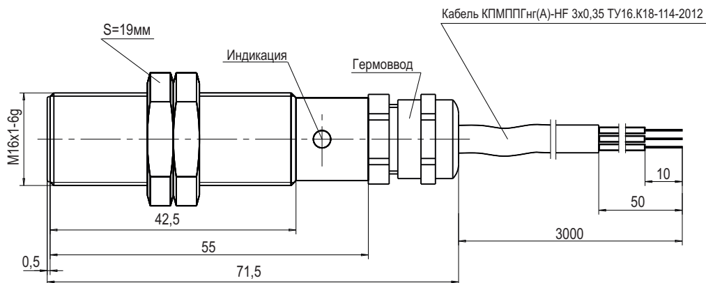
Габаритный чертеж
