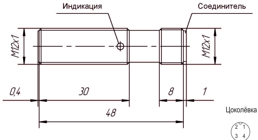
Габаритный чертеж
