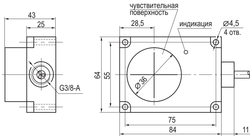
Габаритный чертеж
