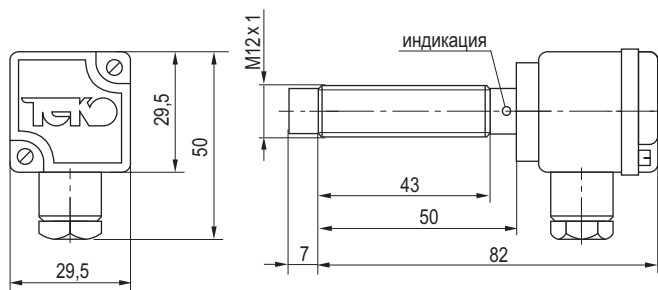
Габаритный чертеж
