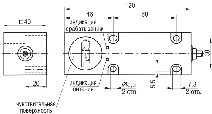
Габаритный чертеж
