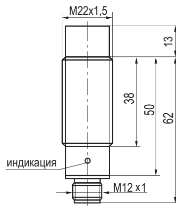
Габаритный чертеж
