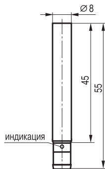
Габаритный чертеж
