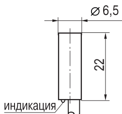
Габаритный чертеж
