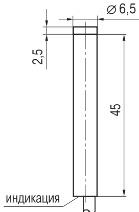
Габаритный чертеж
