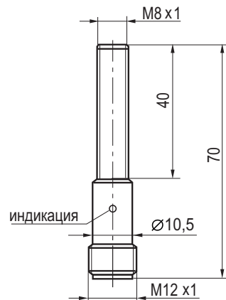
Габаритный чертеж
