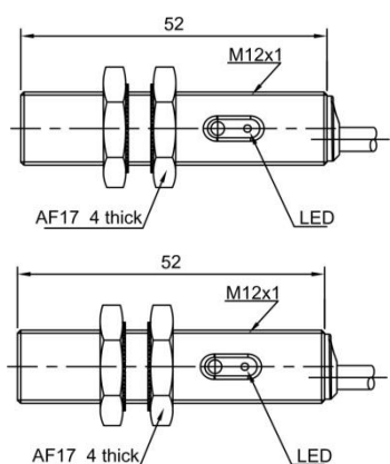
Emitter
