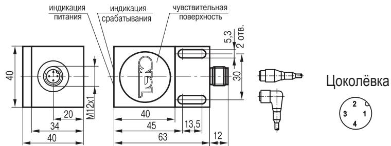
Габаритный чертеж
