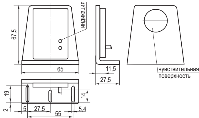
Габаритный чертеж
