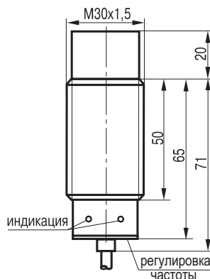
Габаритный чертеж
