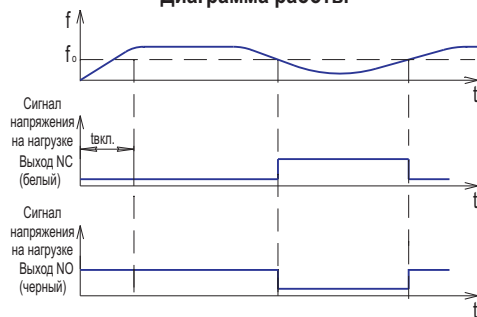
Диаграмма работы
