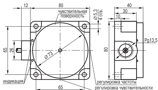
Габаритный чертеж
