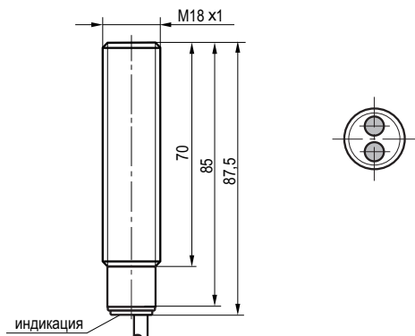
Габаритный чертеж
