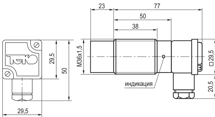
Габаритный чертеж
