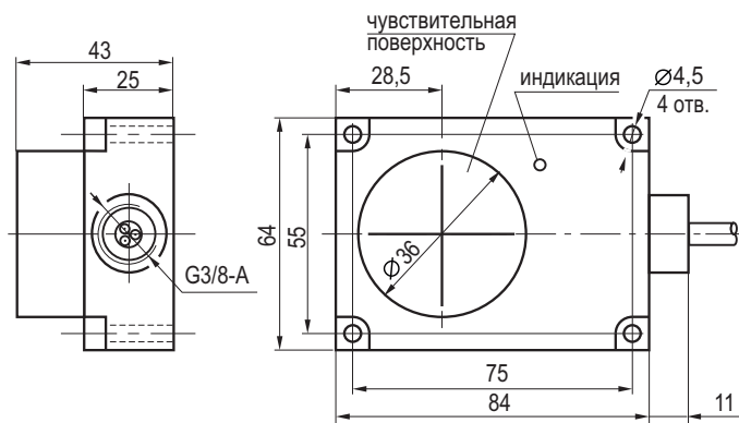
Габаритный чертеж
