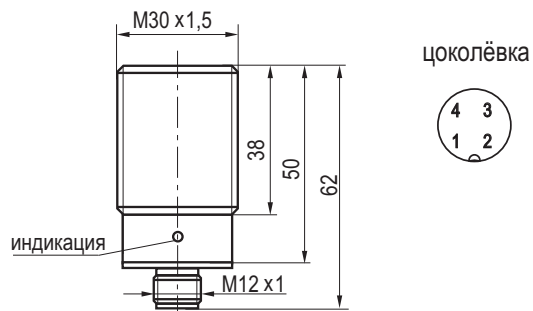
Габаритный чертеж
