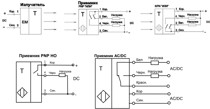
Рис. 1. Схемы подключения Цифрами указаны номера контактов для исполнений с разъемом или клеммником. Положение контактов реле показано при наличии питания и отсутствии объекта воздействия.
