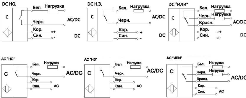
Рисунок 4 - Схемы подключения
