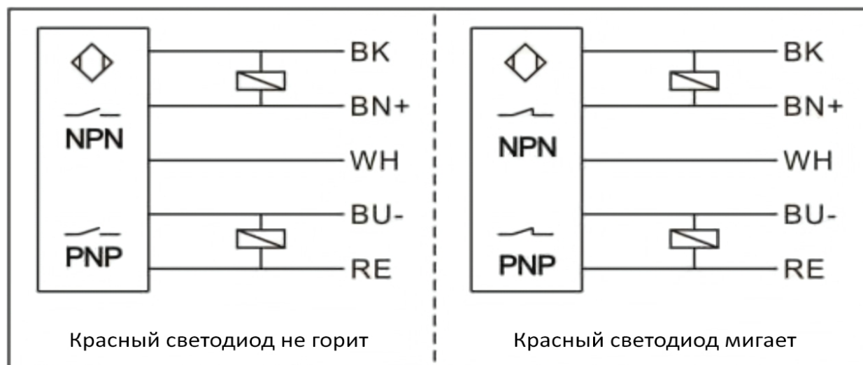
Схема подключения
