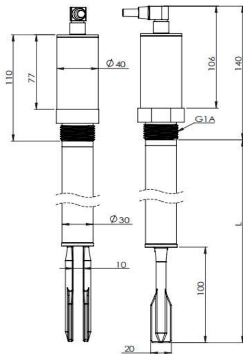
Размеры, мм
