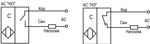
Рисунок 2 – Схемы подключения
