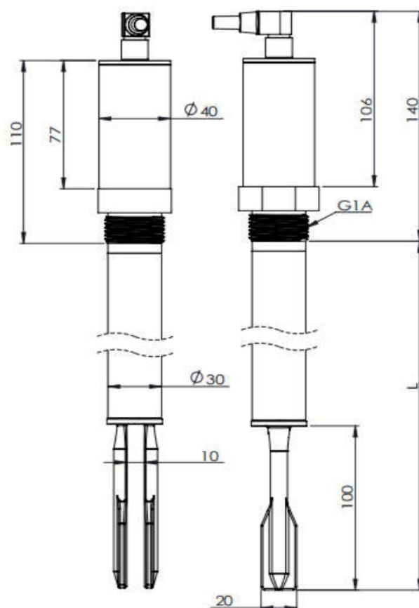
Размеры, мм
