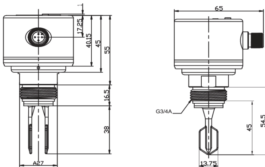
Размеры, мм
