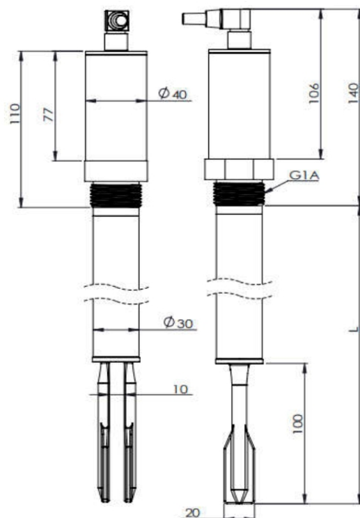
Размеры, мм
