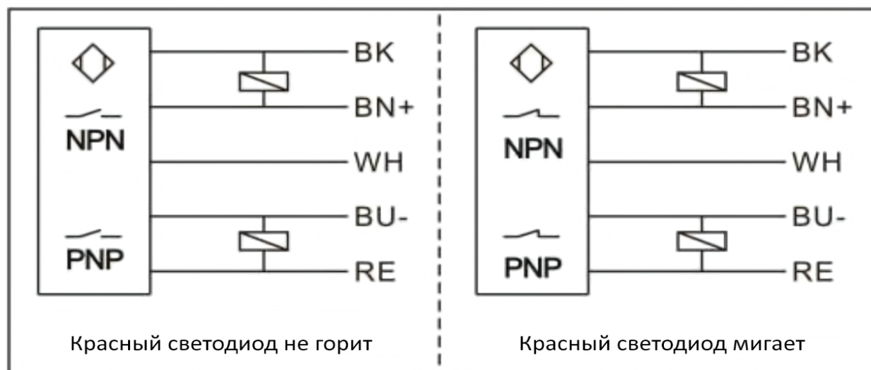
Схема подключения
